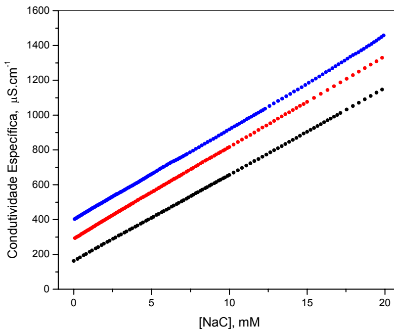
Figura 12: Perfil de condutividade específica versus [\text{NaCl}] na ausência ( \bullet ), e em presença de 20 ( \bullet ) e 100 mM ( \bullet ) de PEO.
