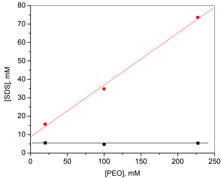
Figura 16: Variação da cac (●) e do psp (●) em função da [PEO] para o sistema SDS-PEO.
