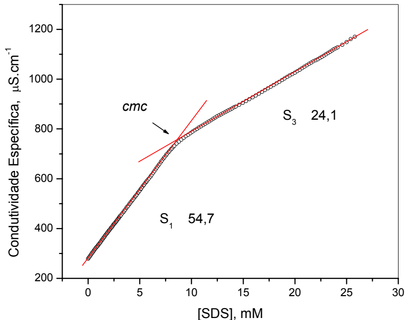
Figura 09: Gráfico de condutividade específica versus [SDS].
