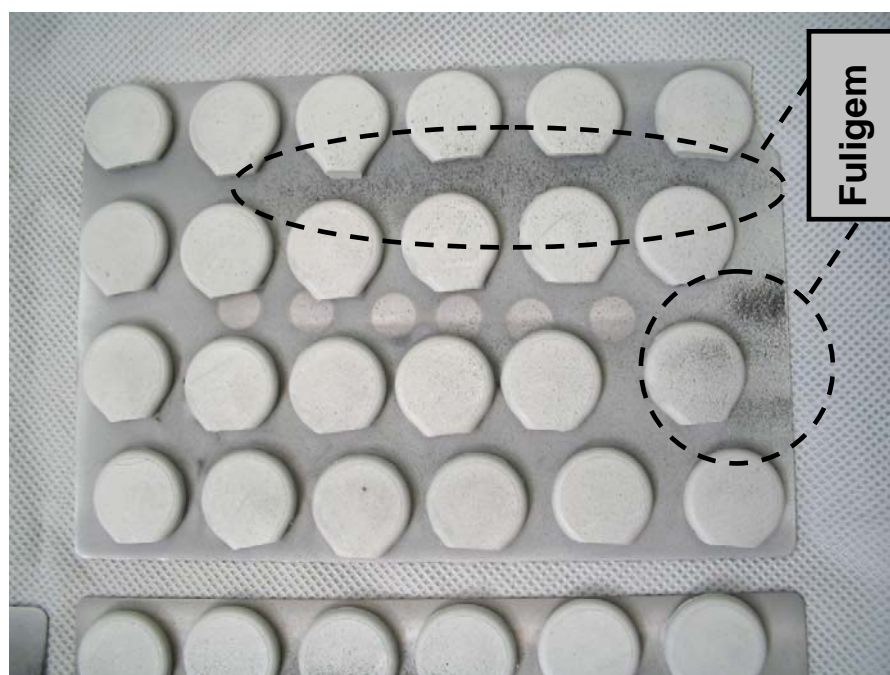
Figura 4.29 - Fuligem depositada no ciclo a 0,5 °C/min.
