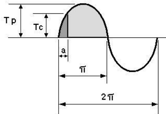
Figura 3.14 - Controle de potência pelo sistema ângulo de fase. T_p – tensão de pico; T_c – valor instantâneo da tensão no momento do corte; a – ângulo de fase no qual é feito o corte pelo disparo do gatilho do tiristor.
