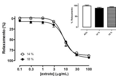
Figura 10: Relaxamento vascular induzido pelos ESO de C. glaziovii contendo 14 % e 18 % de droga. Concentrações crescentes dos extratos (0,1 a 100 µg/mL) foram adicionadas em anéis de aorta de ratos com endotélio intacto contraídos com fenilefrina (1 µmol/L) ( n= 6 ). Inset: Comparação entre os relaxamentos máximos induzidos por 100 µg/mL dos extratos de C. glaziovii contendo 14 e 18% de droga com aquele induzido por acetilcolina (ACh; 1 µmol/L). As barras representam a média \pm EPM do percentual máximo de relaxamento obtido em pelo menos 5 diferentes experimentos.
