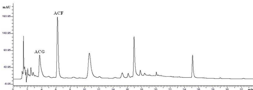
Figura 5: Cromatograma da solução extrativa com 12 % de droga, etanol 30 % (V/V) e 8 dias de maceração: coluna HPLC 150x4,6 mm Zorbax C 18 . Fase móvel em sistema gradiente de ACN e CH 3 COOH 1% fluxo 1,0 mL/min, detecção a 330 nm com detector UV
