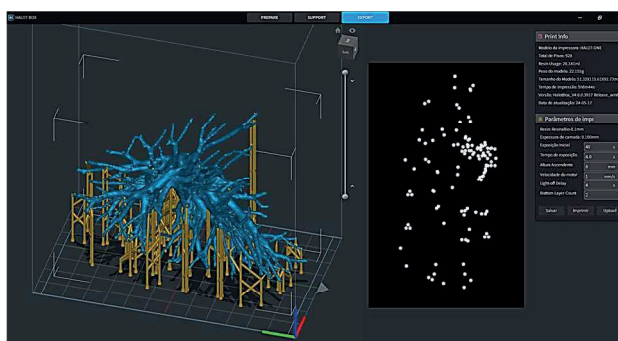
Fig. 9: Fatiamento de um dos conjuntos de brônquios, com os suportes de impressão.
