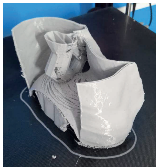
Figura 7: Um dos pulmões sendo impresso em PLA cor cinza, com os suportes de impressão na parte inferior e interna.
